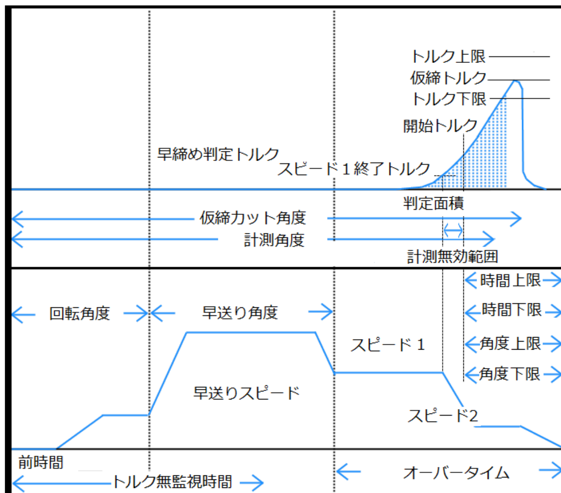
仮締め参考波形
