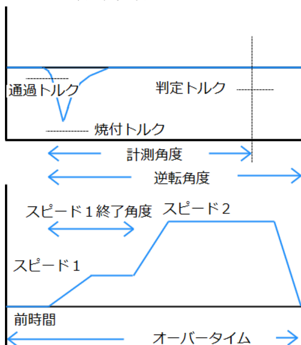
逆転工程参考波形
