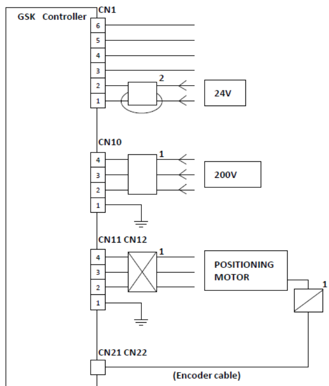
【POSITIONING CONTROLLER】
