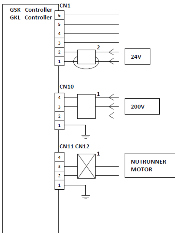
【NUTRUNNER CONTROLLER】
