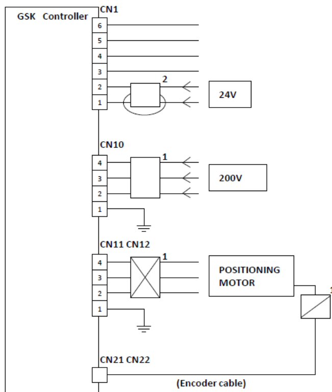
【POSITIONING CONTROLLER】
